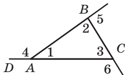
Рис. 146. Внешний угол 4 равен сумме углов 2 и 3
