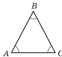
Рис. 86. К признаку равностороннего треугольника
