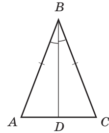
Рис. 83. Луч BD — биссектриса угла B
