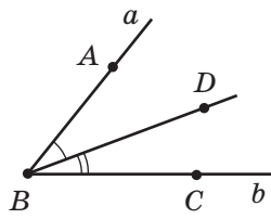
Рис. 18. Луч BD делит угол ABC на два угла
