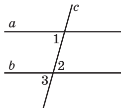
Рис. 121. \angle 1 = \angle 3 , тогда a \parallel b
