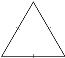
Рис. 82. Равносторонний треугольник
