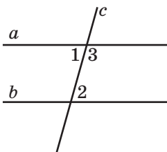
Рис. 120. \angle 2 + \angle 3 = 180^\circ , тогда a \parallel b
