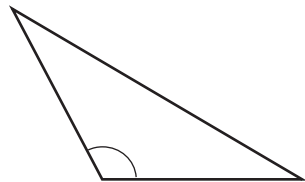
Тупоугольный
