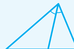
Биссектриса
