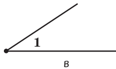
Рис. 17. Обозначение угла
