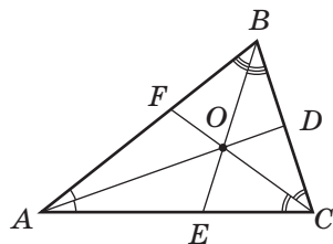
Рис. 187. Точка O — точка пересечения биссектрис треугольника ABC
