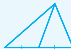
Медиана
