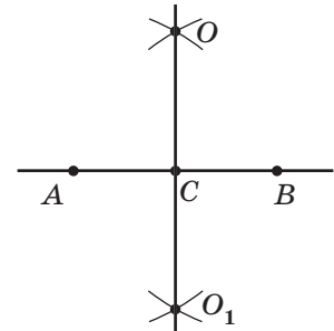
Рис. 172. Построение середины отрезка
