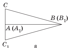
Рис. 107. Прикладывание треугольника A_1B_1C_1 к треугольнику ABC
