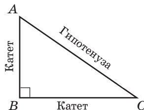
Рис. 147. Прямоугольный треугольник
