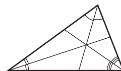
Рис. 98. Три биссектрисы треугольника пересекаются в одной точке
