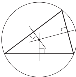
Внутри треугольника
