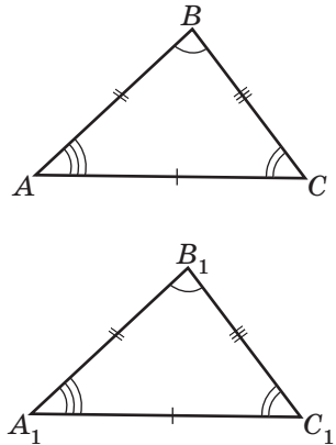
Рис. 56. Треугольники ABC и A_1B_1C_1 равны
