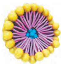
Рис. 34.2. Мицелла ПАВ с гидрофобным веществом внутри
