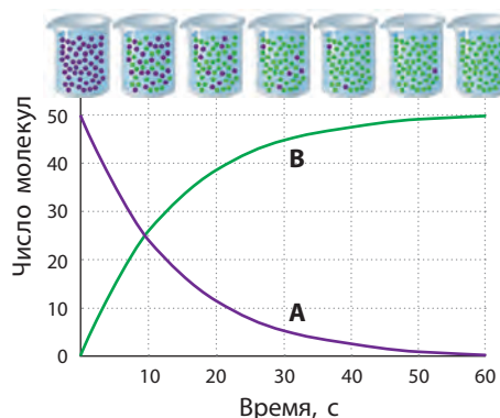
Рис. 20.1. Изменение числа молекул реагента (А) и продукта реакции (В) во время химической реакции (фиолетовым цветом обозначены данные о реагентах, зеленым — о продуктах реакции)
