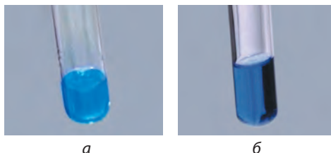
Рис. 36.2. Качественная реакция на глюкозу: а — свежесожденный купрум(II) гидроксид; б — при наличии глюкозы осадок исчезает, образуется соединение темного-синего цвета
