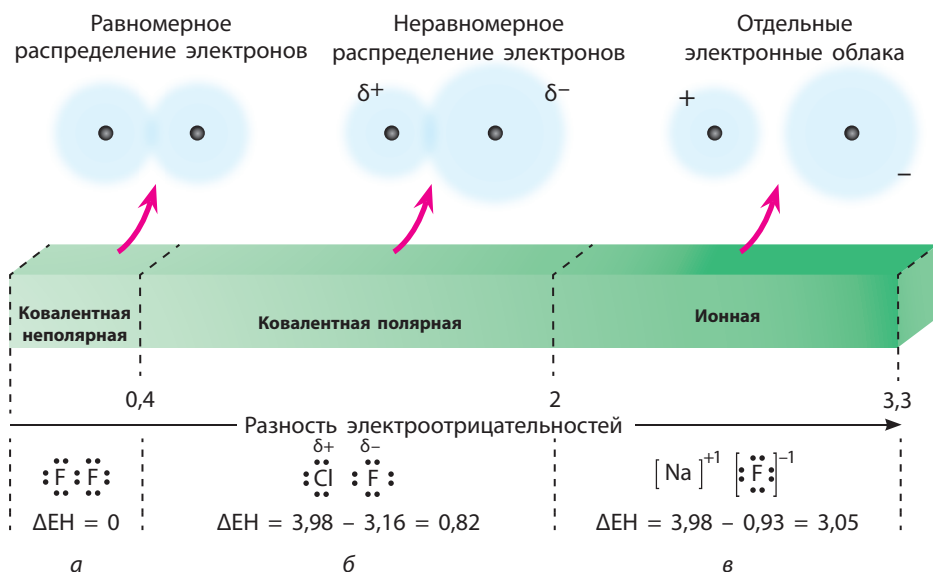
Рис. 2.1. Зависимость типа связи от разности электроотрицательности элементов: a — ковалентная неполярная; б — ковалентная полярная; в — ионная
