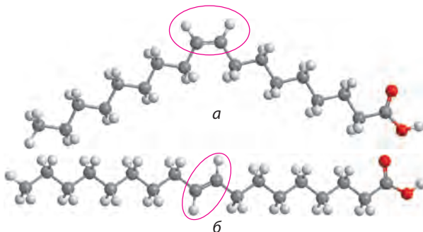
Рис. 35.3. Различные формы олеиновой кислоты: a — цис -форма (естественная); б — транс -форма (модифицированная)
