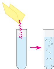
Рис. 20.6. При обычных условиях водород пероксида почти не разлагается (слева), но при добавлении катализатора — марганца(IV) оксида — реакция ускоряется так, что жидкость почти закипает от количества выделяемого кислорода (справа)
