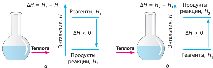
Рис. 18.4. Изменение энthalпии системы при экзотермической (а) и эндотермической (б) реакциях
