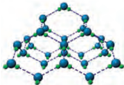
Рис. 5.2. Кристаллические решетки твердой воды: каждая молекула образует по четыре водородные связи с соседними молекулами
