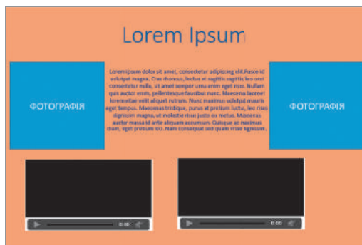
Рис. 11.77. Відображення відеофайлів
