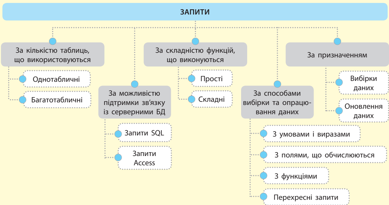
Рис. 3.1. Класифікація запитів
