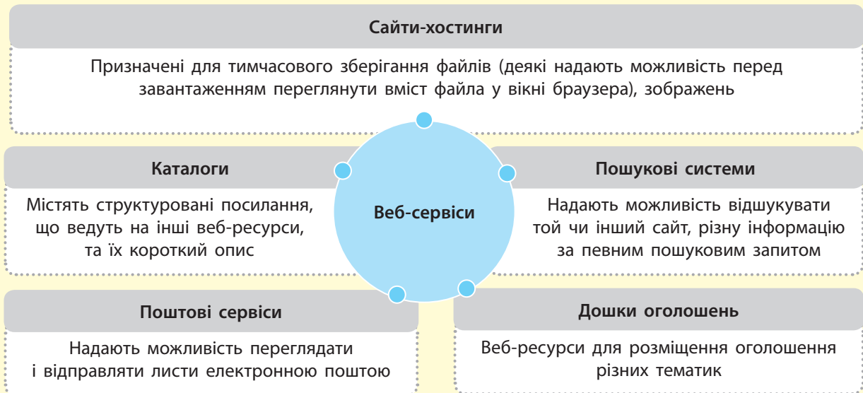
Рис. 11.14. Класифікація веб-сервісів
