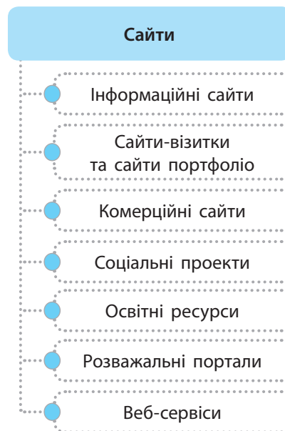
Рис. 11.11. Класифікація сайтів
