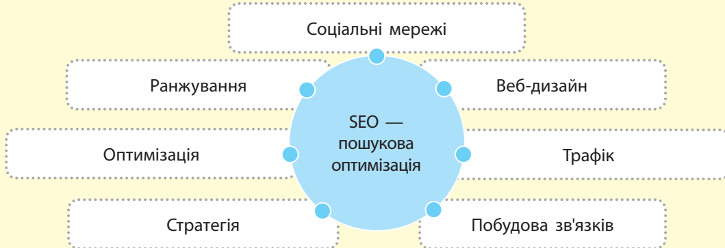
Рис. 11.95. Складові SEO
