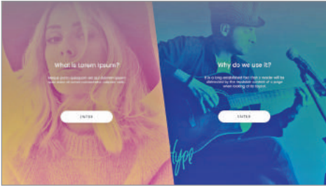
Рис. 11.8. Спліт-екран
