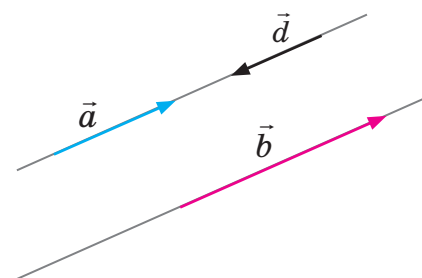
Рис. 10.3. Колінеарні вектори
